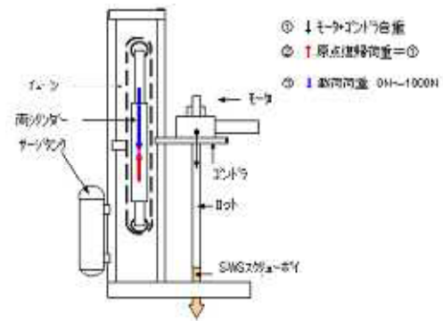
図-1 NSWS 構造および載荷荷重用状態
