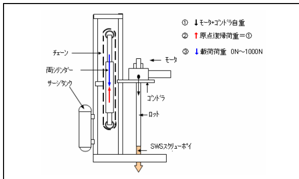
図 - 1 NSWS構造及び載荷荷重作用状態
